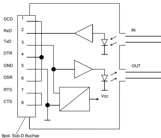
Bild 2 Blockschaltbild
