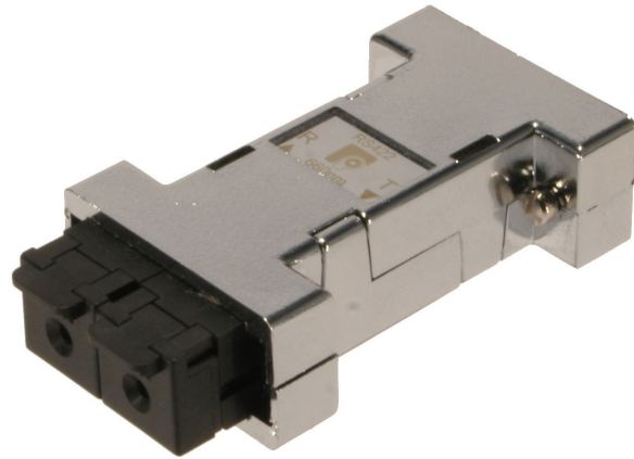
Bild 1 RS232-LWL Interface
