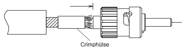
Bild 6 F-ST Steckverbinder mit Crimphülse und Knickschutztülle
