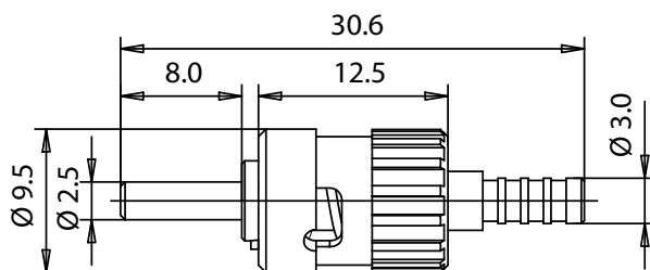
Bild 1 F-ST Steckverbinder
