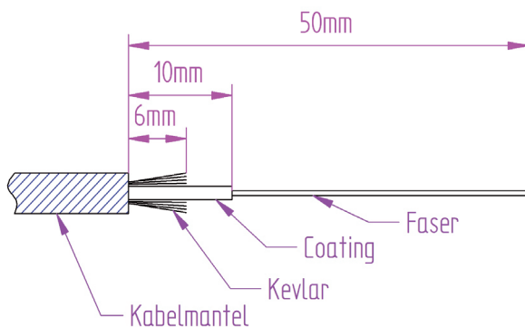
Bild 4 Abisoliermaße am PCF Kabel
