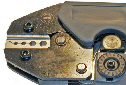
Bild 2 Ausschnitt Crimpgesenk
